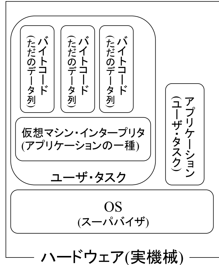
仮想マシン・インタープリタ Process VM
