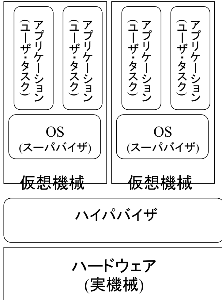
仮想機械 System VM
